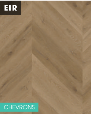
CHEVRONS Prestige Oak Light Amber 152,4 x 1066,8 mm (angle 45°) OFD-055-159
